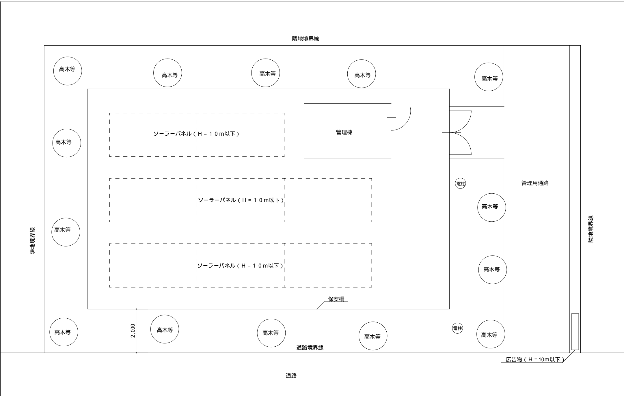
太陽光発電施設景観形成イメージ敷地図
