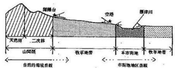
地形の区分
